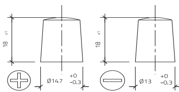
Polausführung 3
