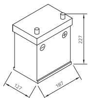
Maße
